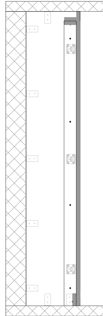
B-B
